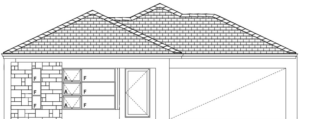
ELEVATION 1 1:100
